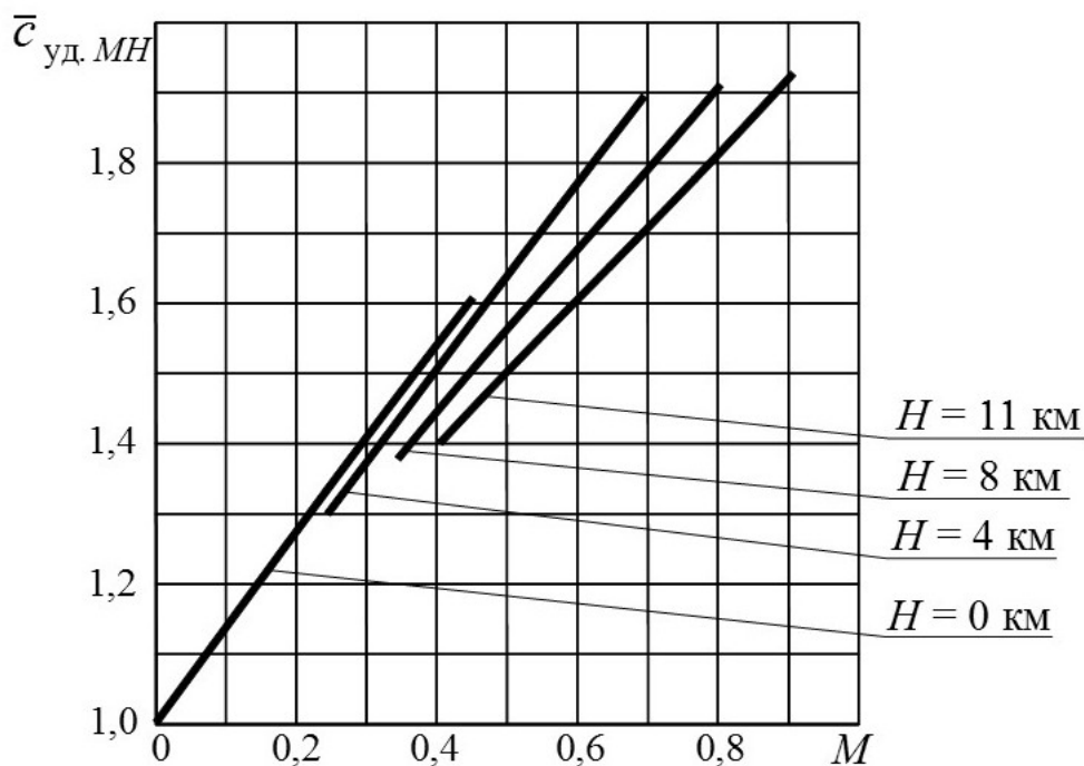
Рис. 2.6. Зависимость относительного удельного часового расхода топлива (для ТРД со степенью двухконтурности m = 4...6 ) от числа M и высоты полета H
