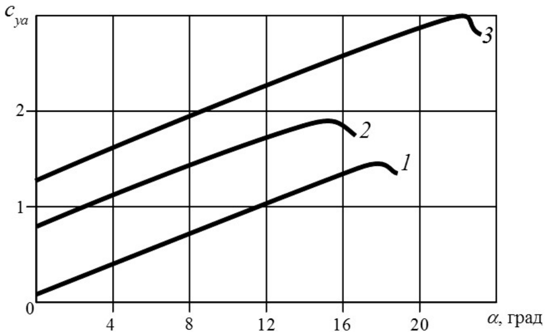
Рис. 3.4. Зависимости коэффициента подъемной силы от угла атаки для самолета 2-го класса с двумя ТРД и следующими геометрическими характеристиками:
