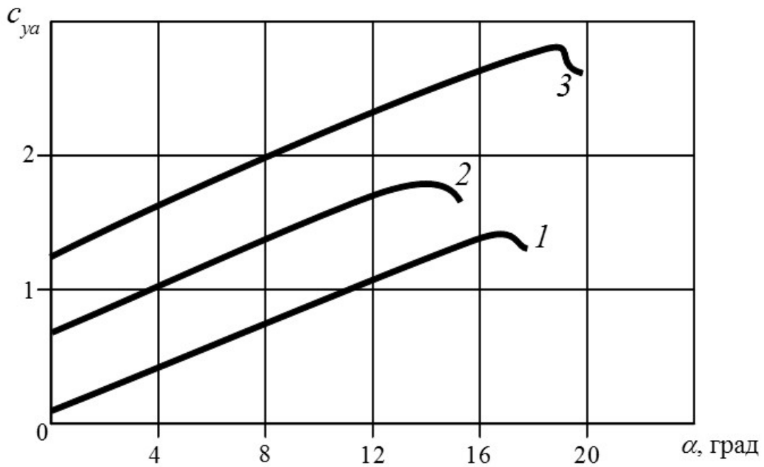
Рис. 3.6. Зависимости коэффициента подъемной силы от угла атаки для самолета 3-го класса с двумя ТРД и следующими геометрическими характеристиками:
