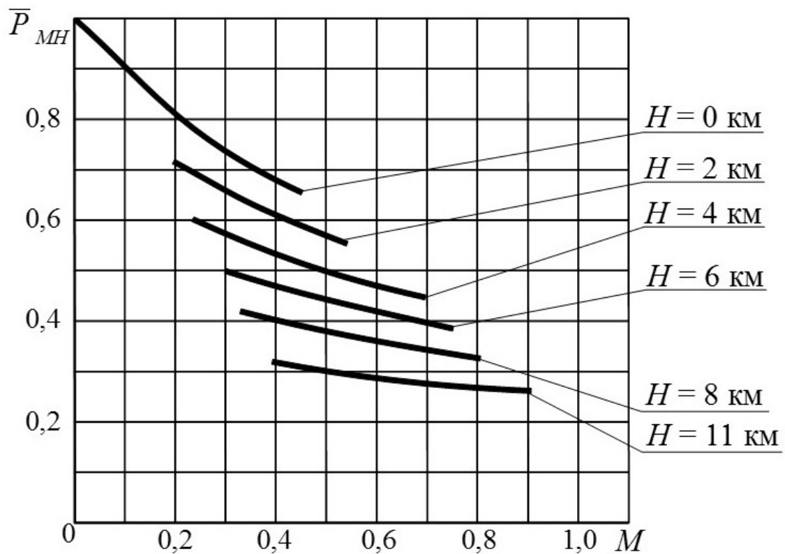
Рис. 2.5. Зависимость относительной тяги (для ТРД со степенью двухконтурности m = 4...6 ) от числа M и высоты полета H
