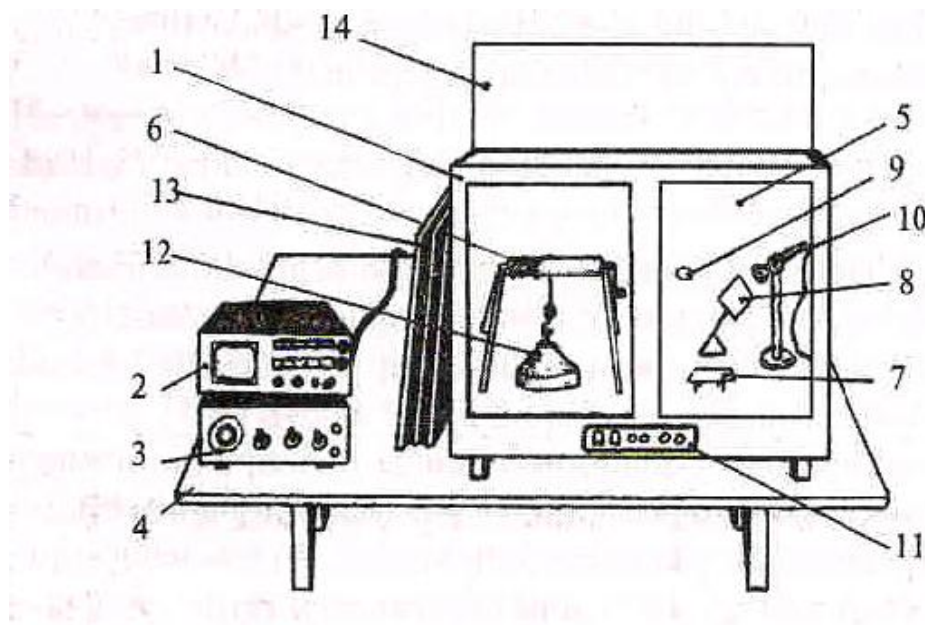
Рис.2.1. Схема лабораторного стенда:
