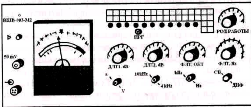
Рис. 2.2. Измеритель шума и вибрации ВШВ-003-М2 (лицевая панель)
