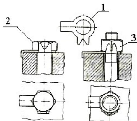
Рис. 2.7. Контровка стопорной шайбой с лапкой:
