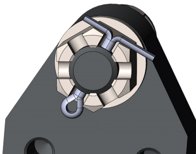
Рис. 2.5. Контровка шплинтами
