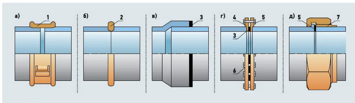
Рис. 2.8 Виды соединения трубопровода:
