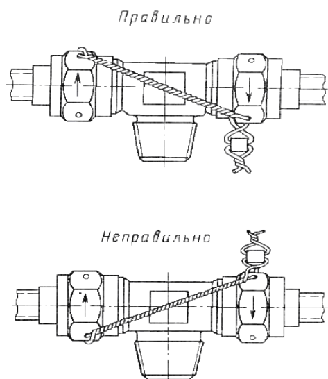
Рис. 2.6. Контровка проволокой
