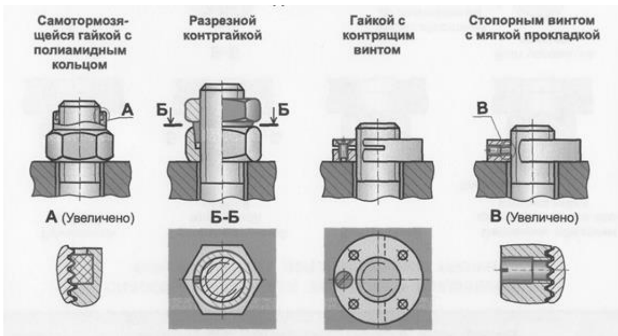
Рис. 2.4. Контровка резьбных соединений
