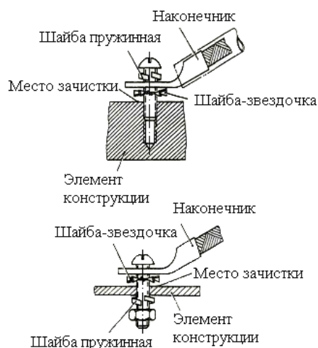
Рис. 5.1. Типовая установка перемычки металлизации
