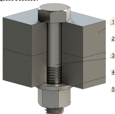
Рис. 2.1. Болтовое соединение:
