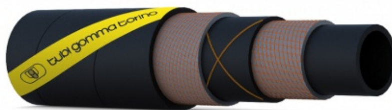
Рис. 2.9. Конструкции рукавов:
