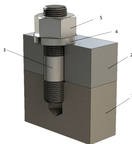
Рис. 2.3. Шпилечное
