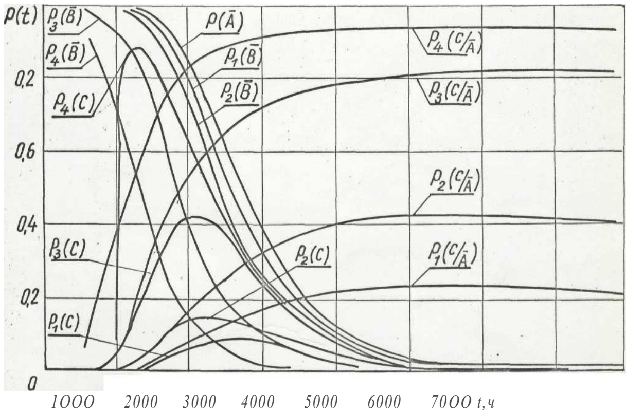
Рис. ПЗ.1. Вероятностные характеристики процесса технической эксплуатации изделий при разных режимах диагностирования и замены для объемного КПД \eta_{\gamma} : 1) при \tau = 100 ч, 2) \tau = 200 ч, 3) \tau = 600 ч, 4) \tau = 1200 ч. \tau
