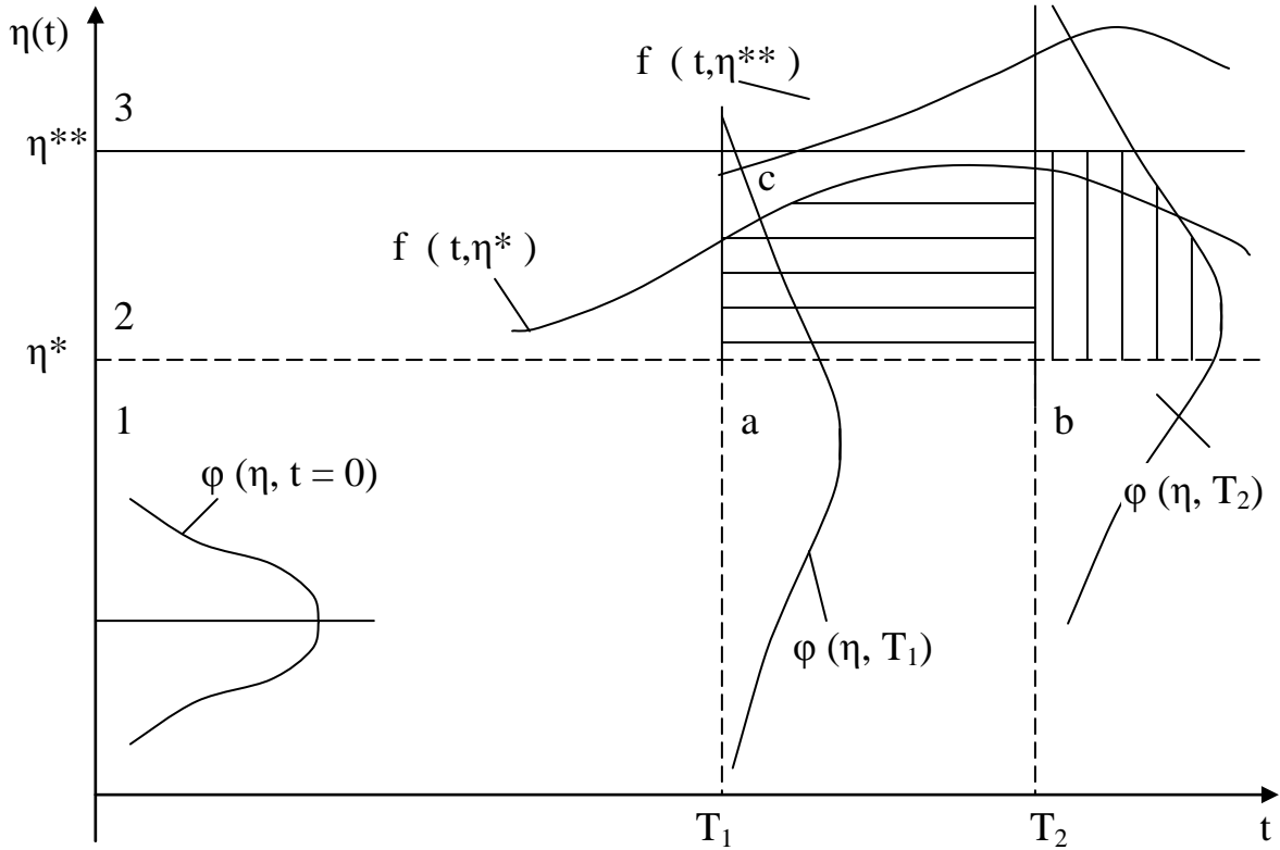
Рис. 4.1. Связь периодических проверок \tau = T_2 - T_1 с упреждающим допуском на диагностический параметр \Delta\eta_i = \eta^{**} - \eta^* (модель экранов).
