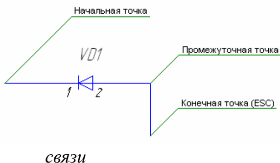
Рисунок 2. Этапы построения линии электрической связи
