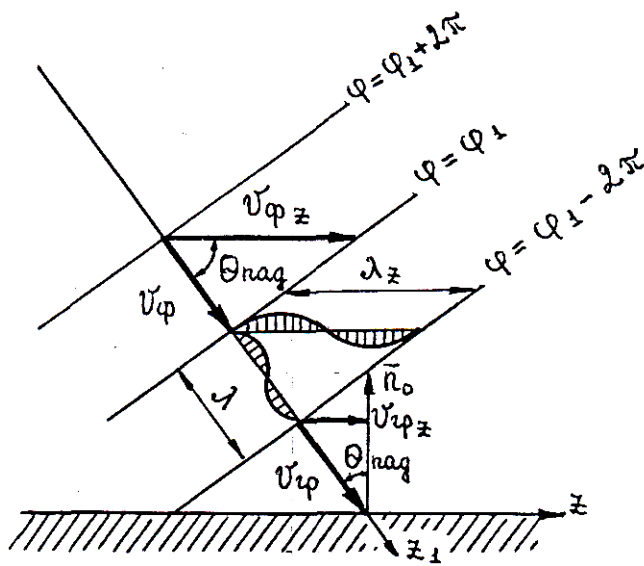
Рис.2.9. Фазовая, групповая скорости и длина волны
