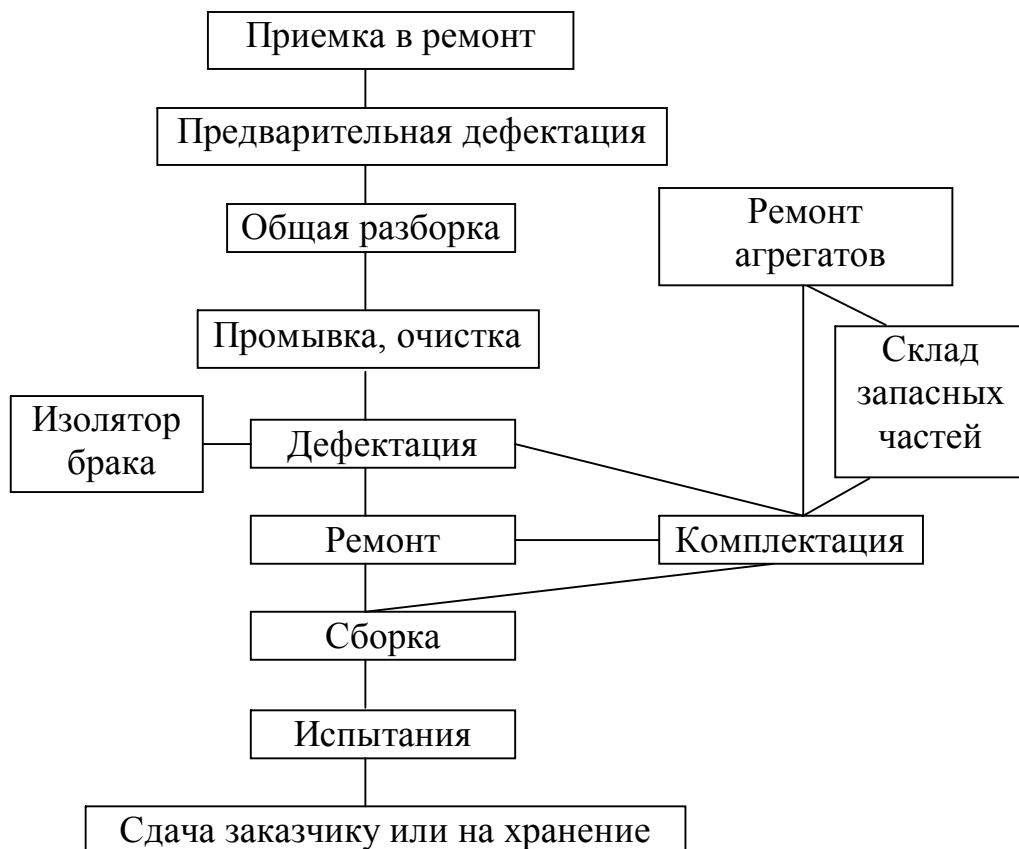
Рис. 1.3. Схема технологического процесса ремонта
