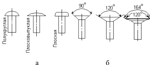
Рис. 3.10. Стержневые заклепки с выступающими и потайными головками:
