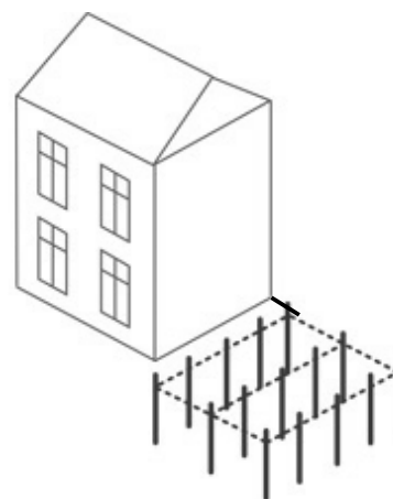
Рис.2. Выносное заземление
