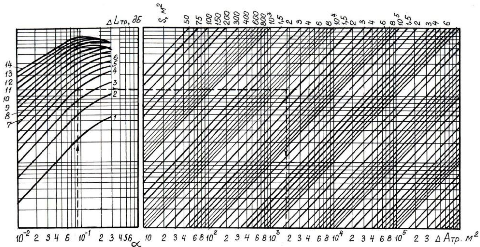
Рис 3.1. Номограммы для расчета \Delta A_{тр}
