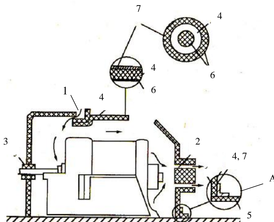
Рис. 2.2. Схема звукоизолирующего кожуха.
