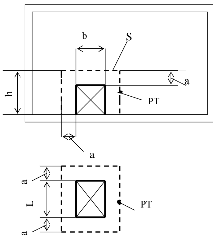
Рис. 2.1. Схема источника шума и расчетной точки
