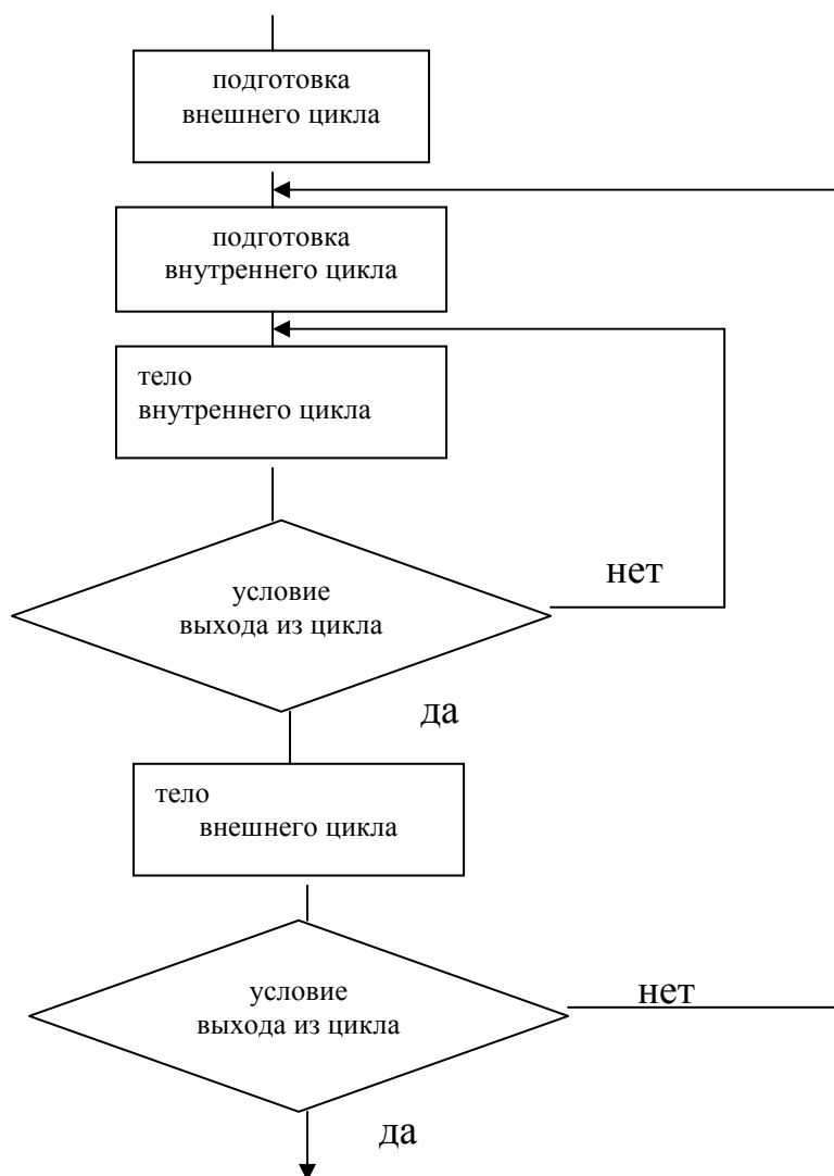
Рисунок 11 Схема алгоритма сложного цикла глубиной два
