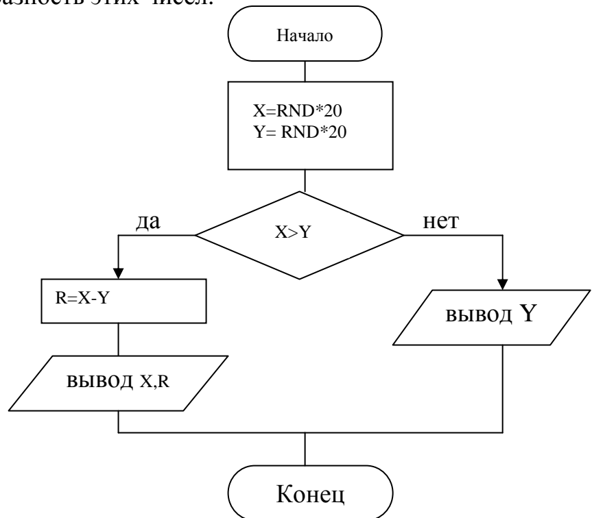
Рисунок 4 Схема алгоритма к примеру 7.1
