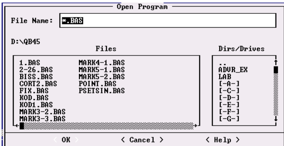
Рисунок 3 Диалоговое окно " Open Program"
