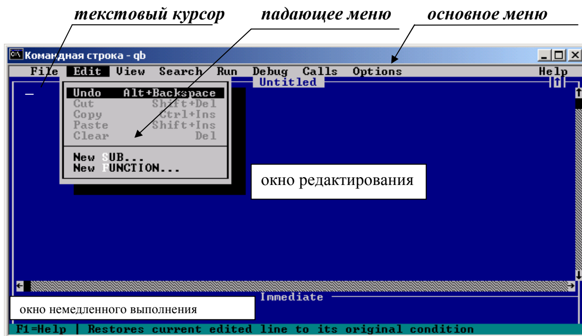
Рисунок 1 - Экран редактора QuickBASIC, версия 4.5
